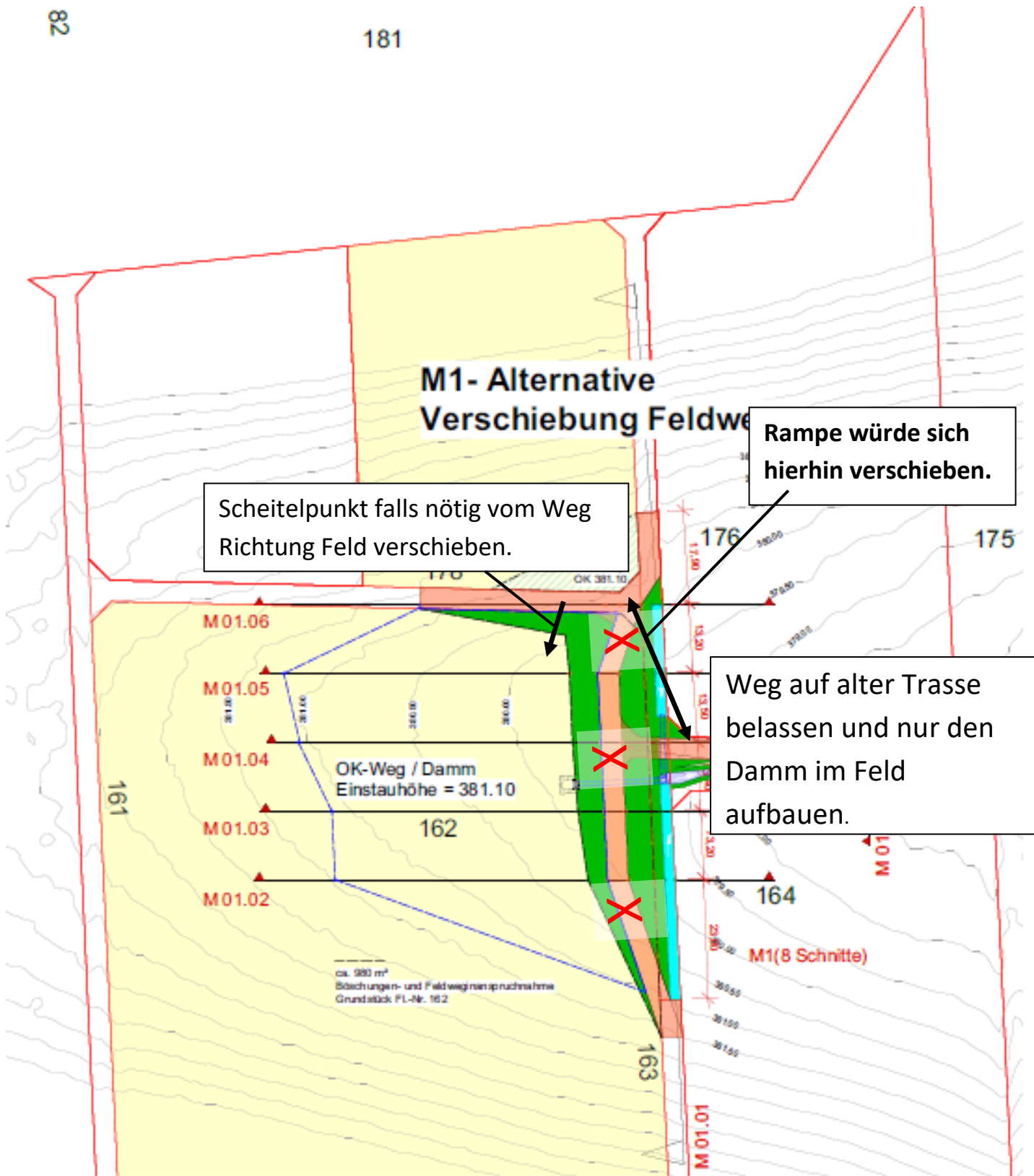
Zeichnung M 1:500
